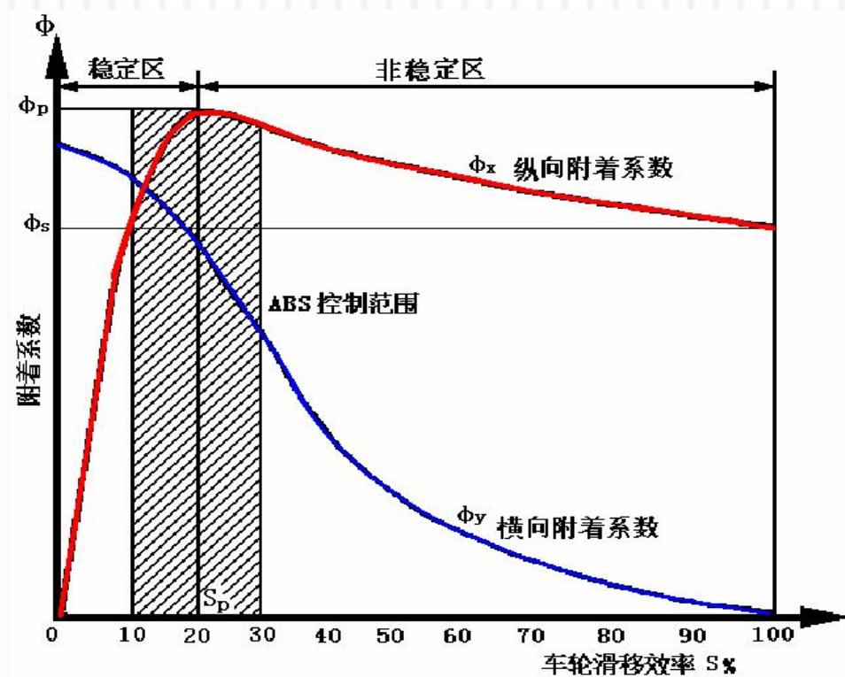
干燥硬实路面附着系数与滑移率的关系
